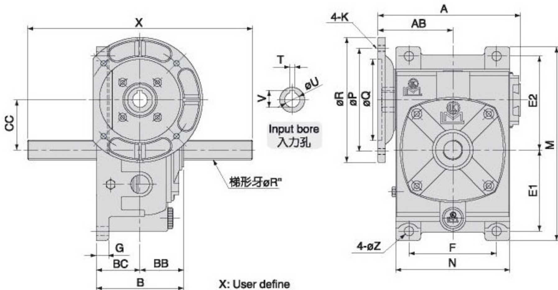
尺寸表 Dimension(m/m)
