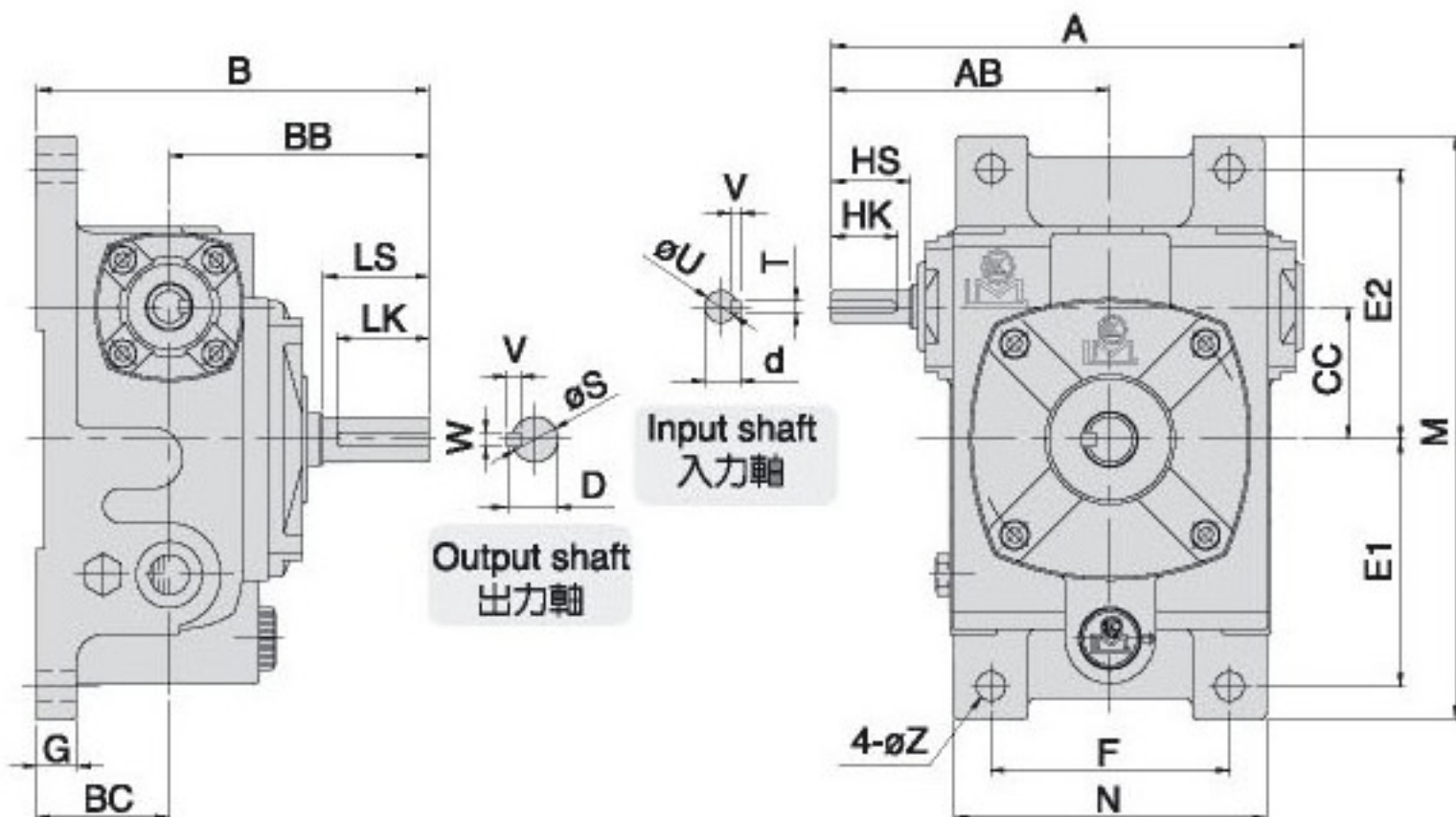
尺寸表 Dimension(m/m)
