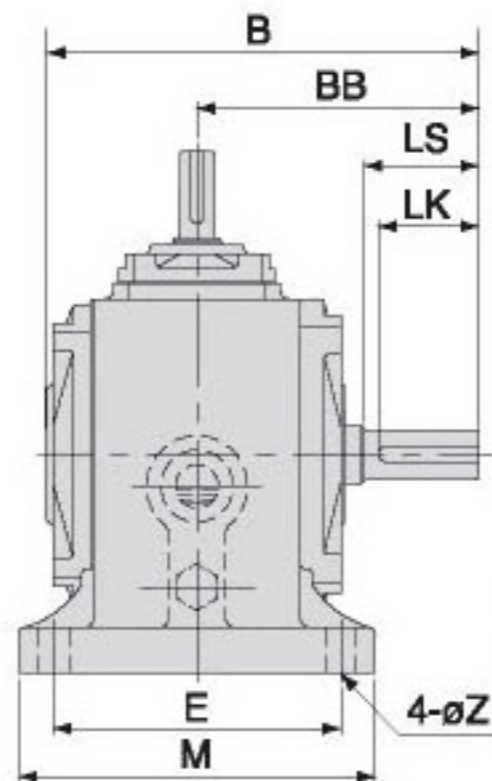
尺寸表 Dimension(m/m)
