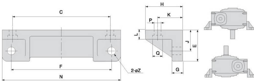
尺寸表 Dimension
