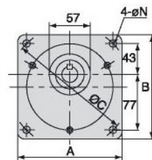
SVDL-A法蘭面 型號Model : 11
