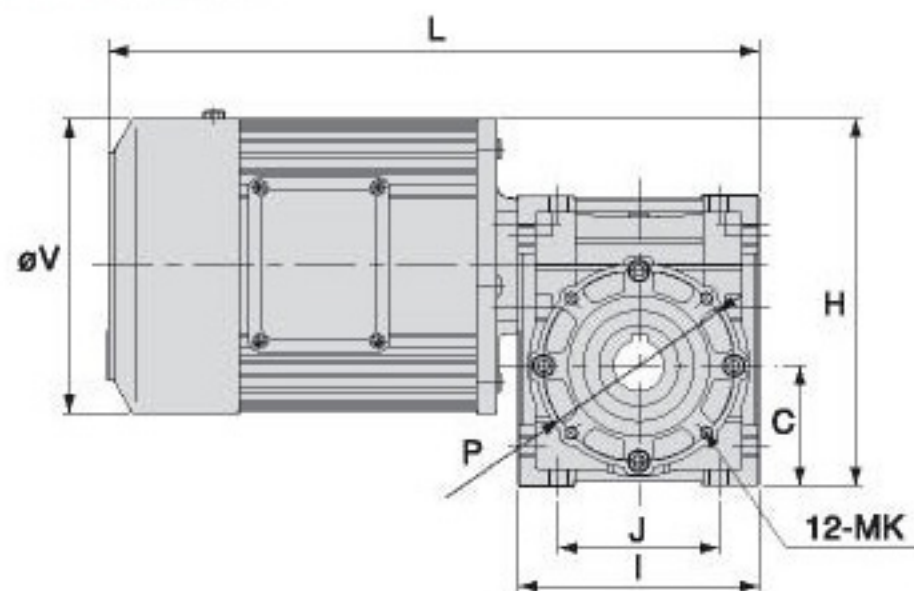
尺寸表 Dimension(m/m)
