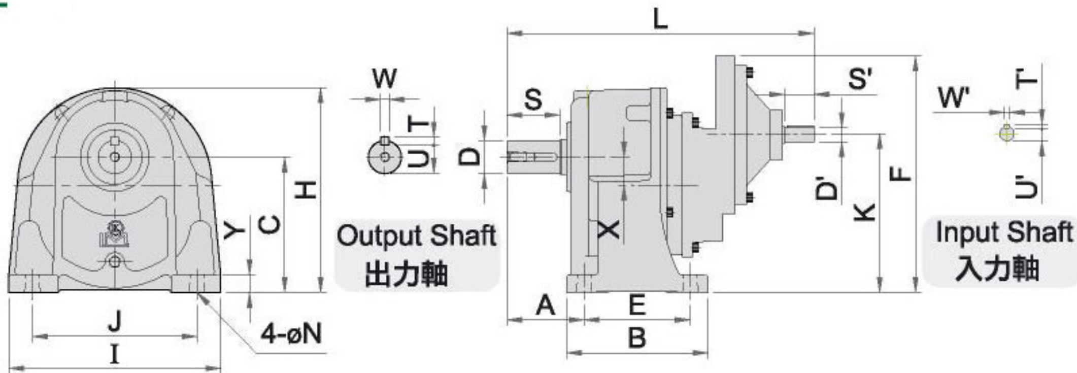
尺寸表 Dimension
