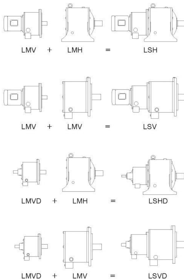
多速比減速機型號速比一覽表（速比超過1/6000以上請另議）（扭距表僅供參考） Model/Speed Ratio Table for Multi-stage Reducer (speed ratio above 1/6000 excluded)
